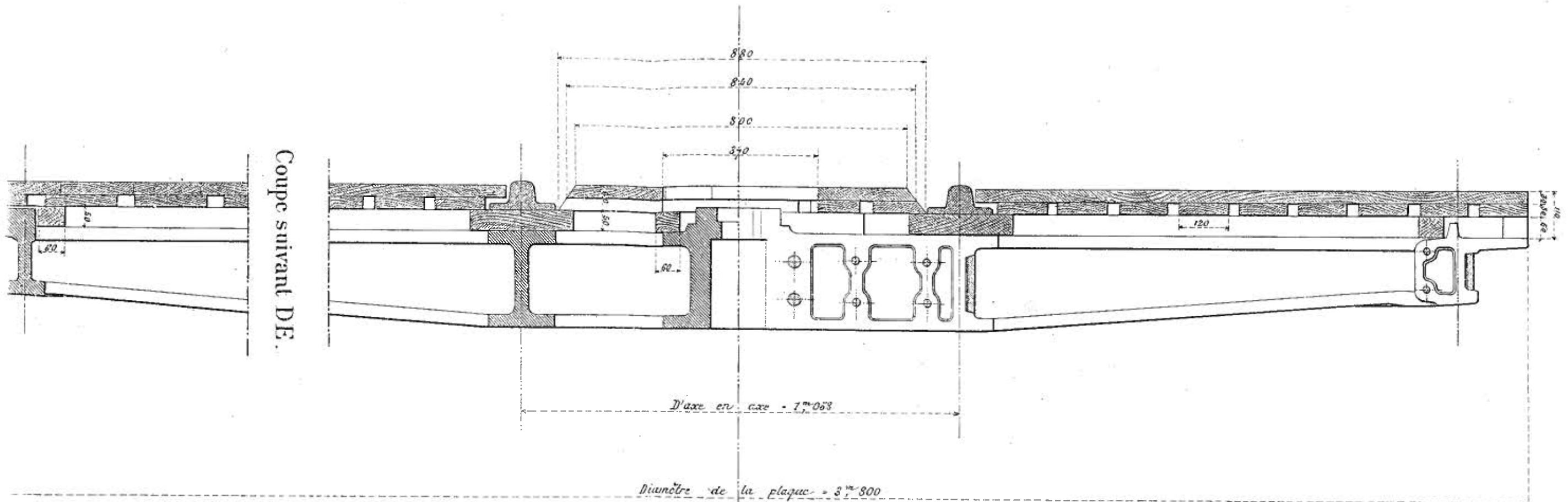
Coupe suivant ABC.
