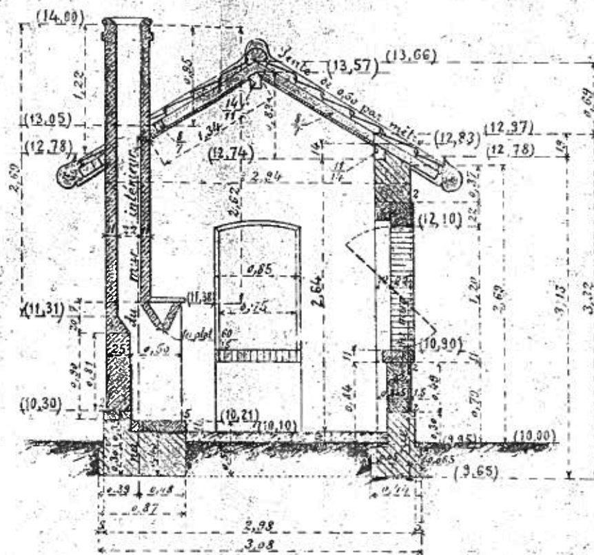
Echelle : — 0 m 02 p r 1 mètre (1/50)
