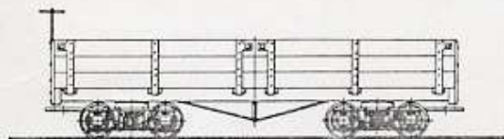
R815 軽便ボギー無蓋車ホト・ORE CAR
