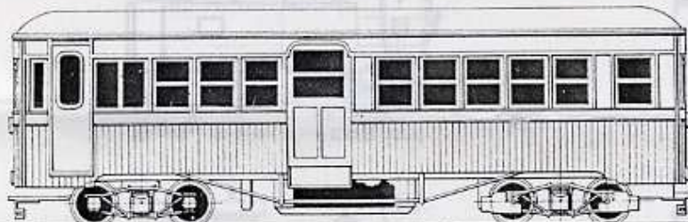
R607 頸城ホジ3・HOJI-3 D.C.
