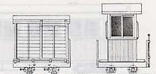
R816 木曾小型貨車 KISO WAGON
