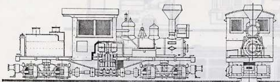
R203 シェイ (クラスA) ・ SHAY CLASS-A 13-2
