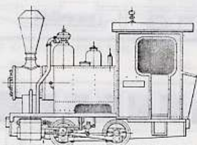
R205 南宮 (5短B型) ・ O-4-OT AMENOMIYA
