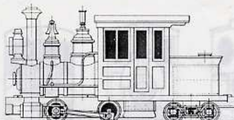
R206 フォーニー・0-4-4T FORNEY
